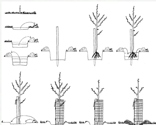
Postup výsadby stromu od vytyčení, až po zamulčování a povýsadbový řez stromu. Poslední dvě činnosti nemusíme provádět přímo při výsadbě na podzim, ale až na jaře, respektive povýsadbový řez v předjaří (od poloviny února do konce března).
